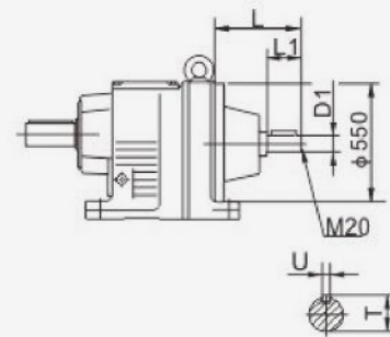
R..167R97(R107)
