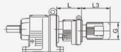
R..167R97(R107)
